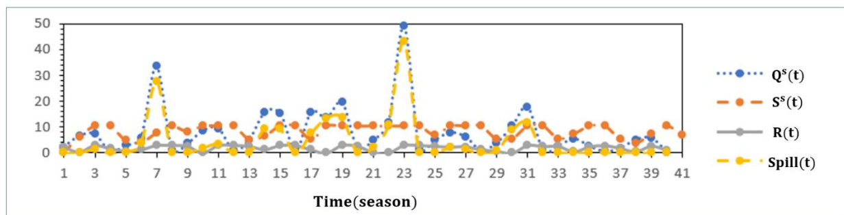
Fig. 8- Inflow, outflow and dam storage volume changes in noncyclic operation (MCM) شکل ۸- تغییرات آورد رودخانه، حجم ذخیره مخزن، رهاسازی عمدی از سد و سرریز از آن در بهره‌برداری غیرسیکلی (م.م.م)
