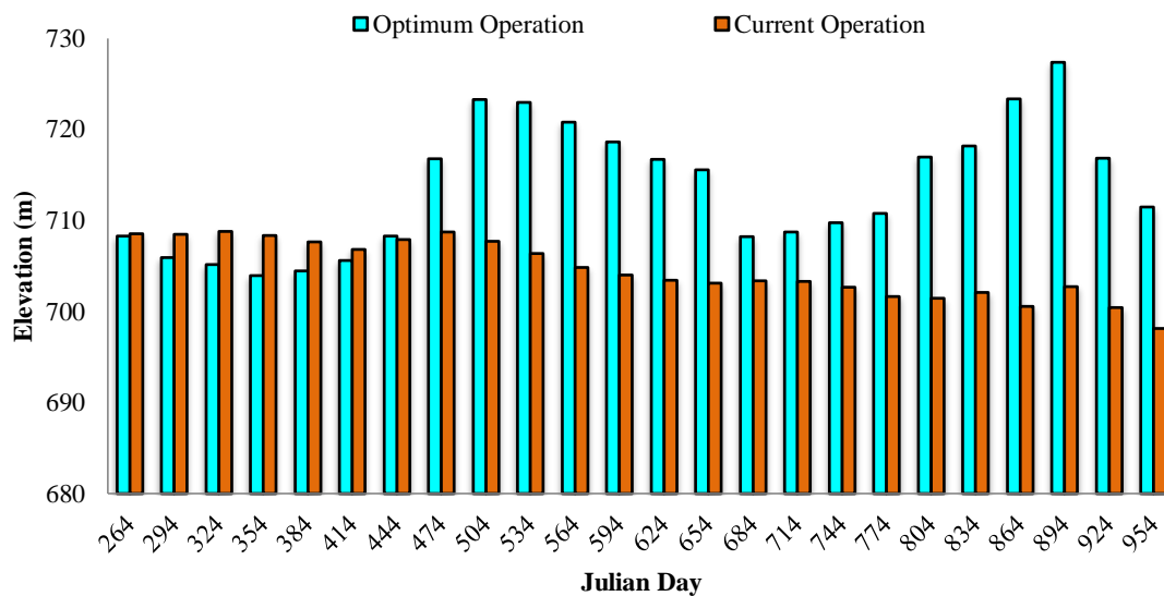
Fig. 16- Reservoir water level during simulation for current condition and optimal policy شکل ۱۶- رقوم سطح آب مخزن در طول دوره شبیه‌سازی به ازای شرایط موجود و سیاست بهینه
