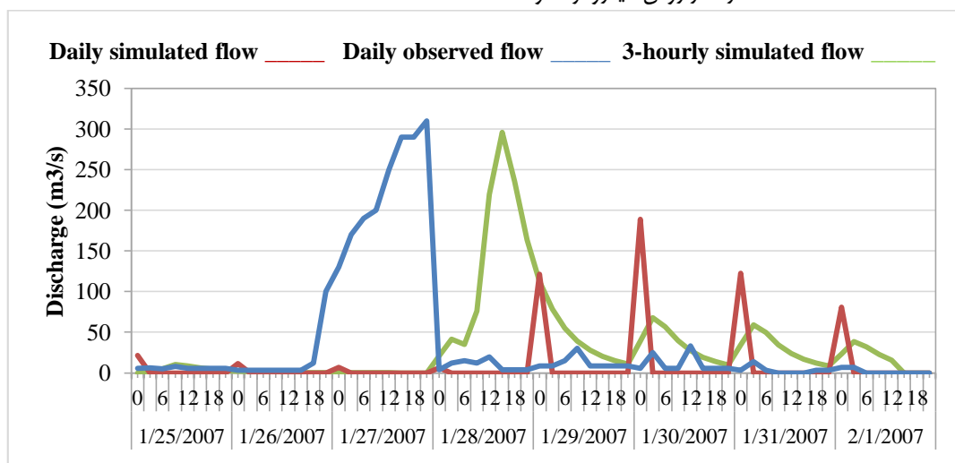
Fig. 8- The results of simulating the flow rate on January 27, 2007 with one-day and 3-hour time steps شکل ۸- نتایج شبیه‌سازی دبی سیلاب رخ داده در ۲۷ ام ژانویه سال ۲۰۰۷ در گام‌های زمانی یک‌روزه و ۳ ساعته
