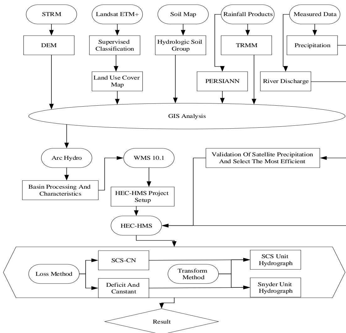
Fig. 1- The flowchart of the method used in this research to simulate the precipitation-runoff process شکل ۱- نمودار گردش روش کار در این مطالعه برای شبیه‌سازی فرآیند بارش-رواناب
