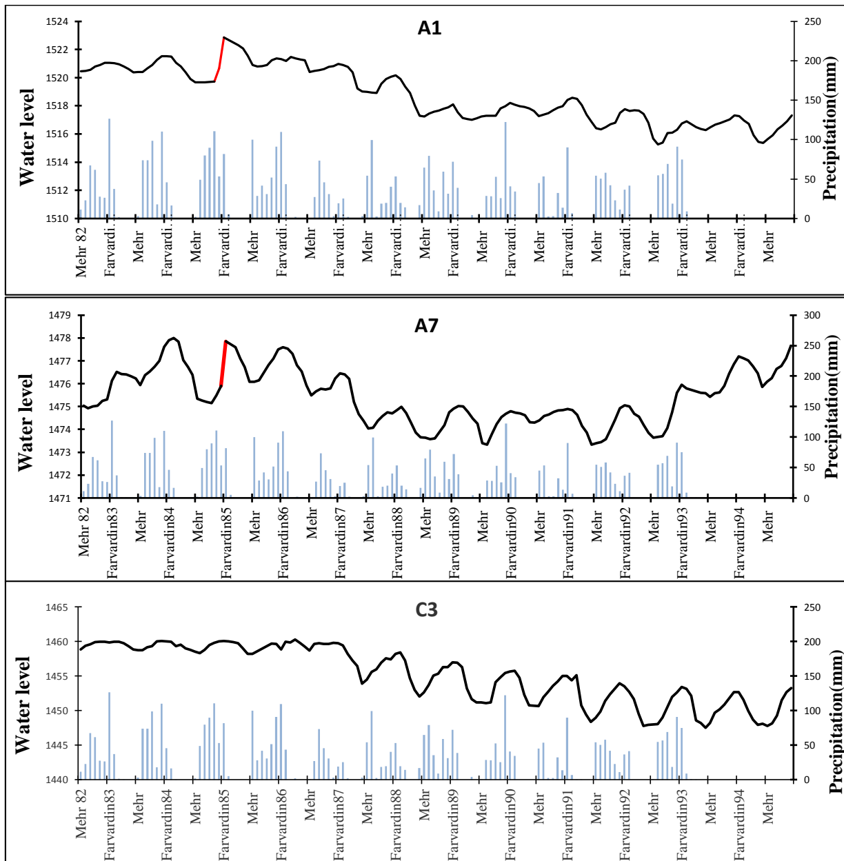
Fig. 7- Hydrographs of the observation wells A1, A7, and C3 during the 12-year survey time شکل ۷- هیدروگراف چاهک‌های مشاهده‌ای A1، A7 و C3 در طول دوره آماری ۱۲ ساله
