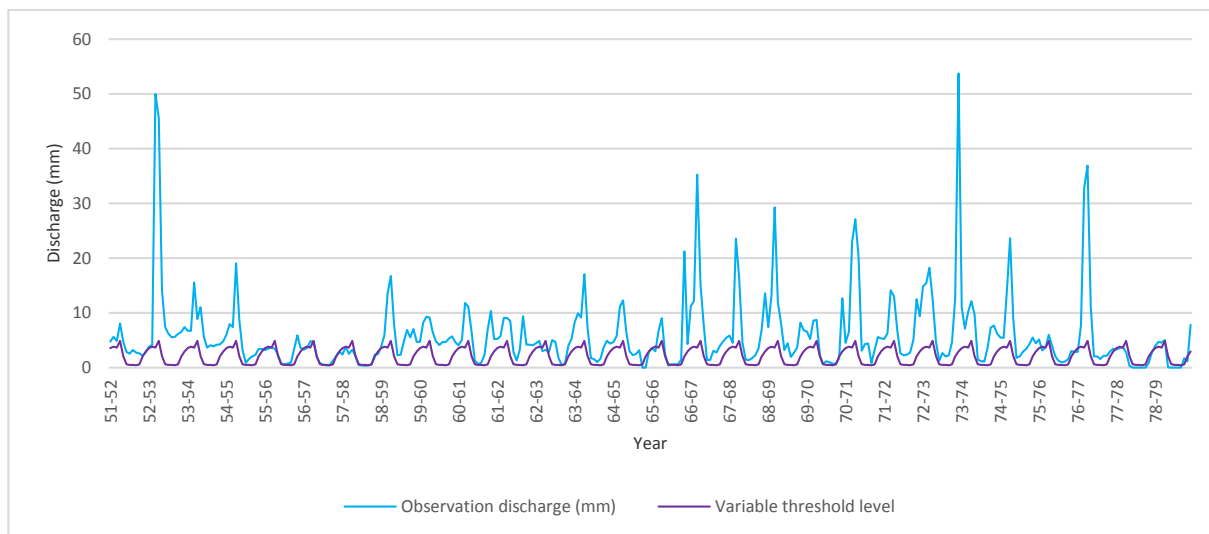
Figure 11: Variable threshold level of the monthly runoff during the undisturbed period شکل ۱۱- سطح آستانه متغیر در مقیاس زمانی ماهانه در دوره دست نخورده
