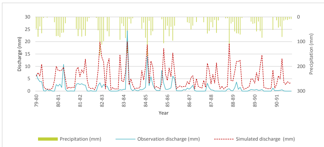
Figure 10: Observation and simulated discharges in disturbed period شکل ۱۰- دبی شبیه‌سازی شده و دبی مشاهداتی در دوره آشفته
