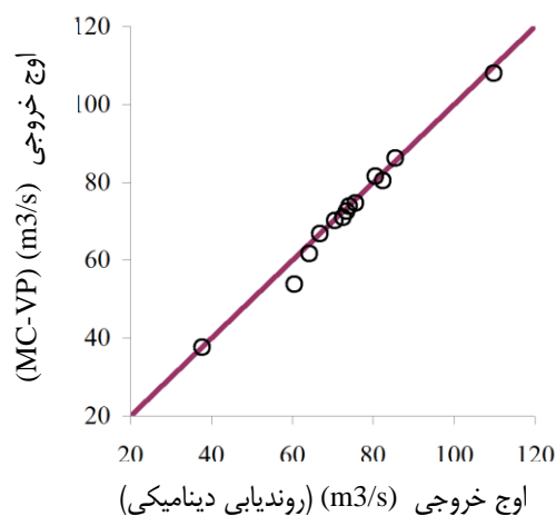
شکل ۸- مقایسه دبی اوج خروجی دو روش روندیابی دینامیکی و MC-VP
