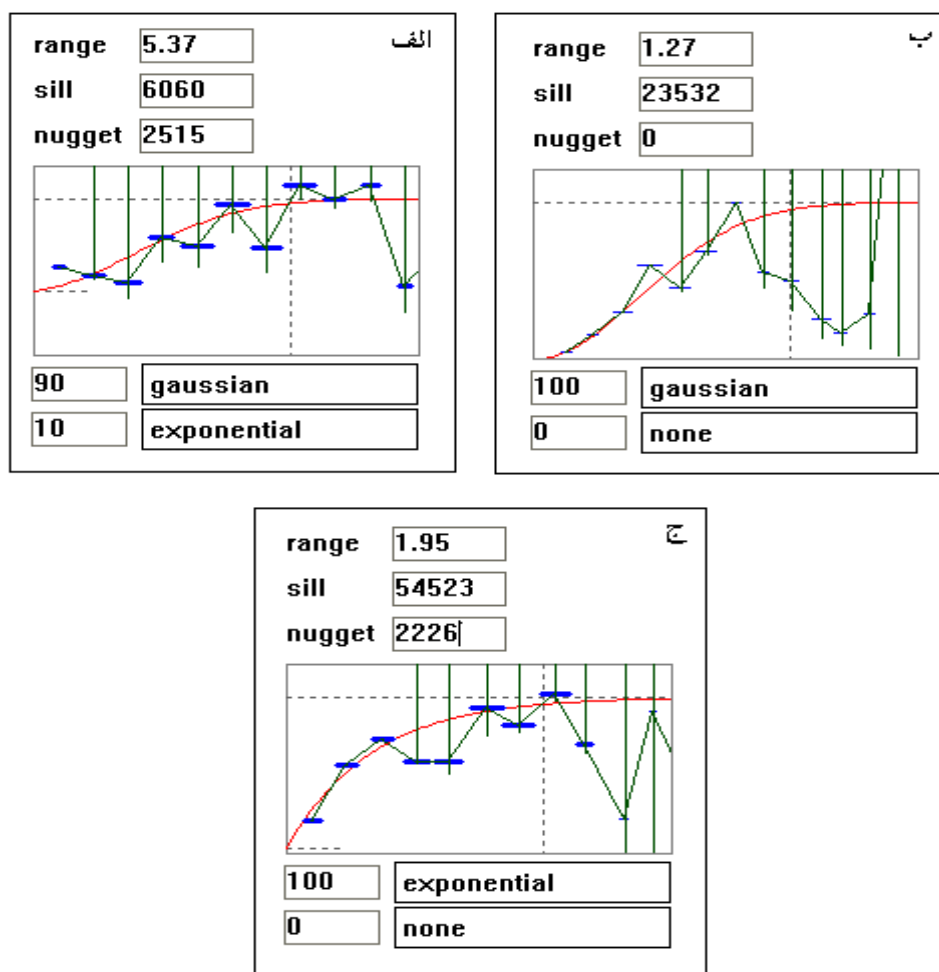
شکل ۵- نیم تعبیرنمای فازی بارندگی سالانه حالت اول در هر یک از مناطق الف) منطقه A (ب) منطقه B (ج) منطقه C.
