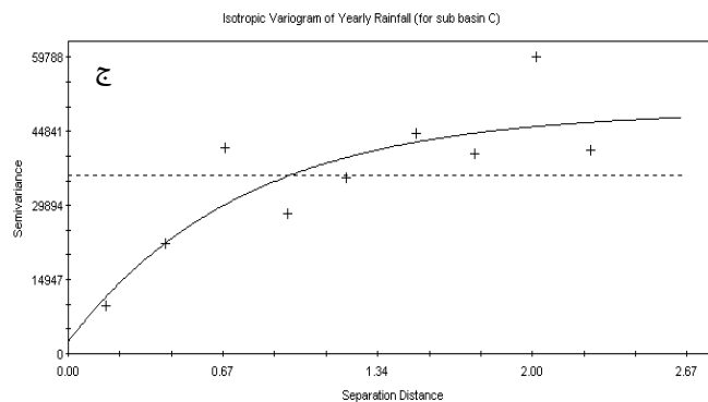
شکل ۴- تغییرنا بارندگی سالانه در هر یک از مناطق تفکیک شده: الف) منطقه A (ب) منطقه B (ج) منطقه C.
