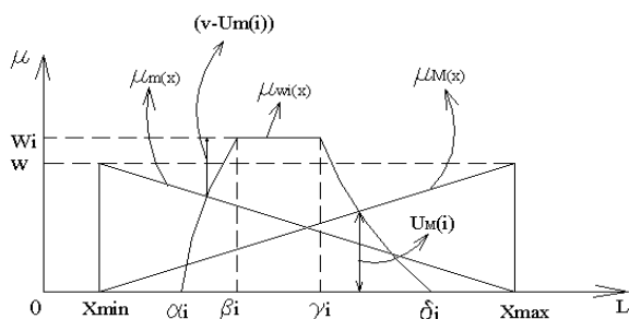
شکل ۲- توابع عضویت مجموعه‌های ماکزیمم و مینیمم
