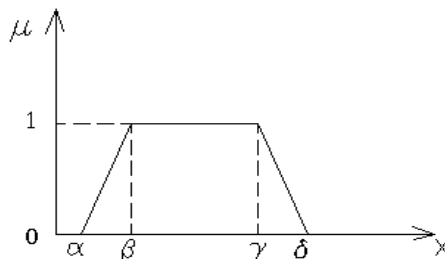
شکل ۱- عدد فازی ذوزنقه‌ای روش مجموعه‌های ماگزیمم و مینیمم
