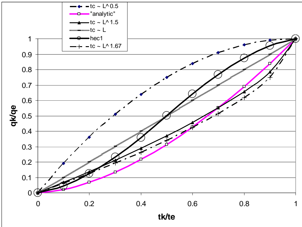
شکل ۵- مقایسه هیدروگراف حاصل از روش‌های مختلف تعیین خطوط همزمان پیمایش و روش تحلیلی موج سینماتیک بر مبنای روش زمان - مساحت
