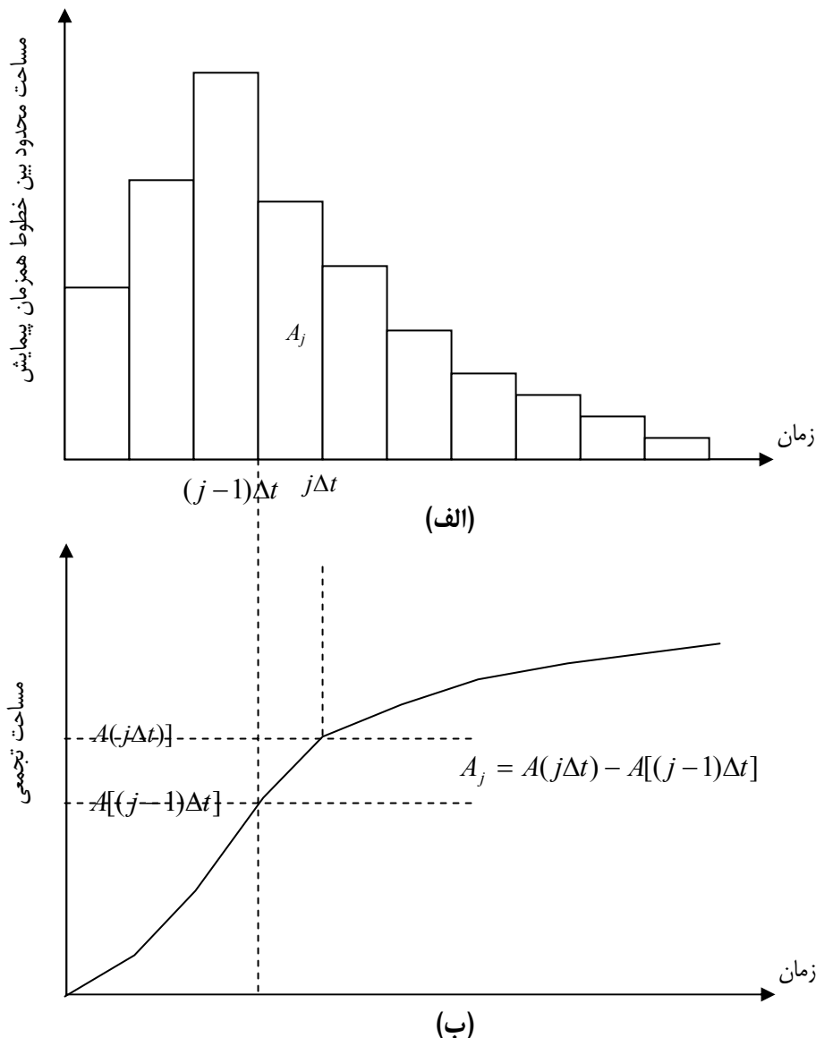
شکل ۲- (الف) هیستوگرام زمان - مساحت و (ب) منحنی تجمعی مساحت (اقتباس از (Maidment 1993))
