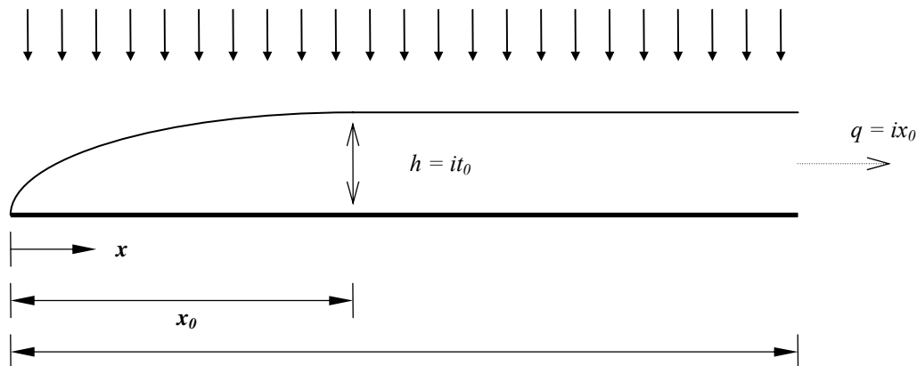
شکل ۳ - پروفیل سطح آب در زمان t=t_0 بر روی صفحه مستطیلی تحت بارش مؤثر به شدت i
