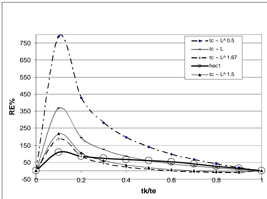
شکل ۶- خطای نسبی روش‌های مختلف تولید هم پیمایش نسبت به روش تحلیلی (موج سینماتیک)
