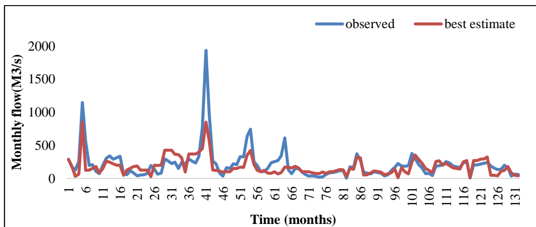
Fig. 8- SWAT validation diagram for the 11-year period (2007-2017) at Mill and Moghan Dam Station شکل ۸- نمودار حاصل از اعتبارسنجی مدل SWAT برای دوره ۱۱ ساله (۲۰۱۷-۲۰۰۷) در ایستگاه سد میل و مغان
