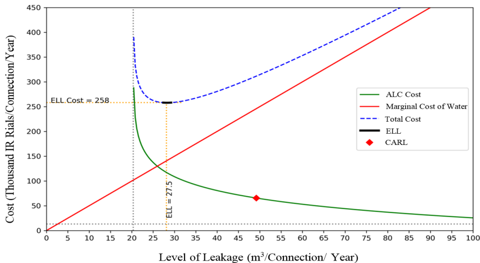
Fig. 7- Analysis of economic level of leakage for district J شکل ۷- تحلیل سطح اقتصادی نشت برای ناحیه J
