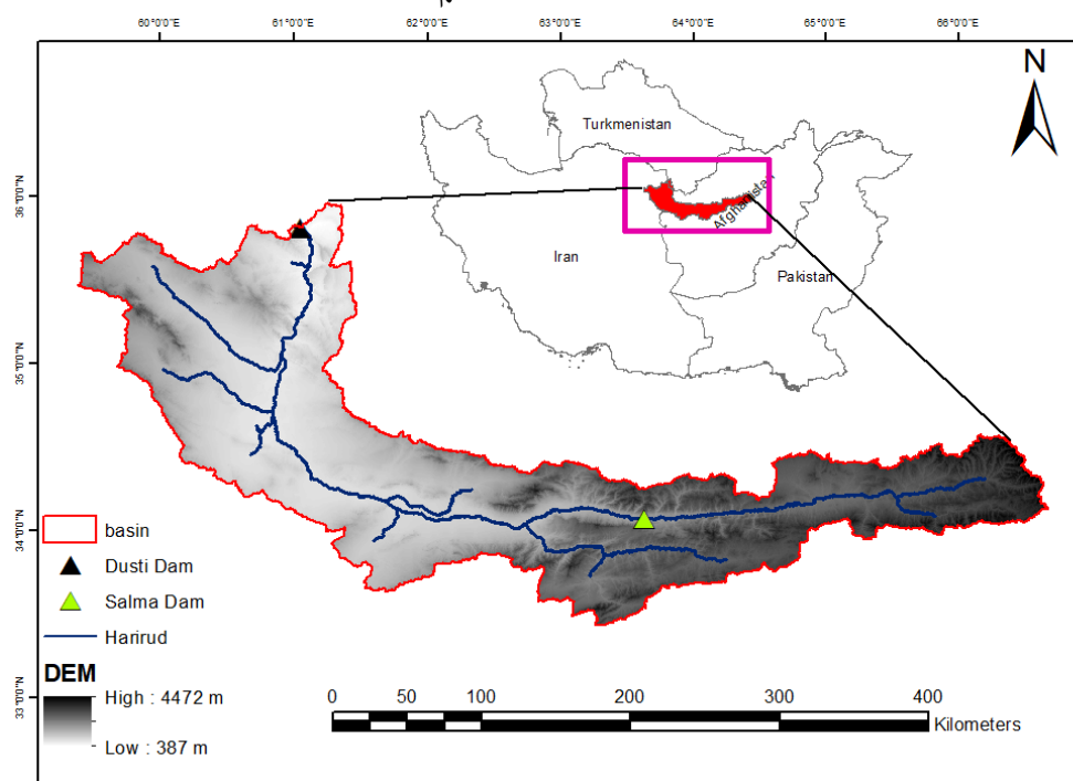
Fig. 1- Location of Dusti river basin, Harirud river, Dusti and Salma dams (DEM Adopted from USGS site) شکل ۱- موقعیت حوضه آبریز سد دوستی، رودخانه هریرود و سد های دوستی و سلما (اطلاعات DEM برگرفته از سایت USGS)
