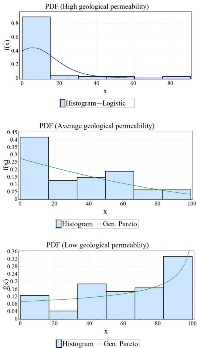
Fig. 5- Probability density function of geological permeability groups شکل ۵- توابع چگالی احتمال گروه‌های نفوذپذیری زمین‌شناسی
