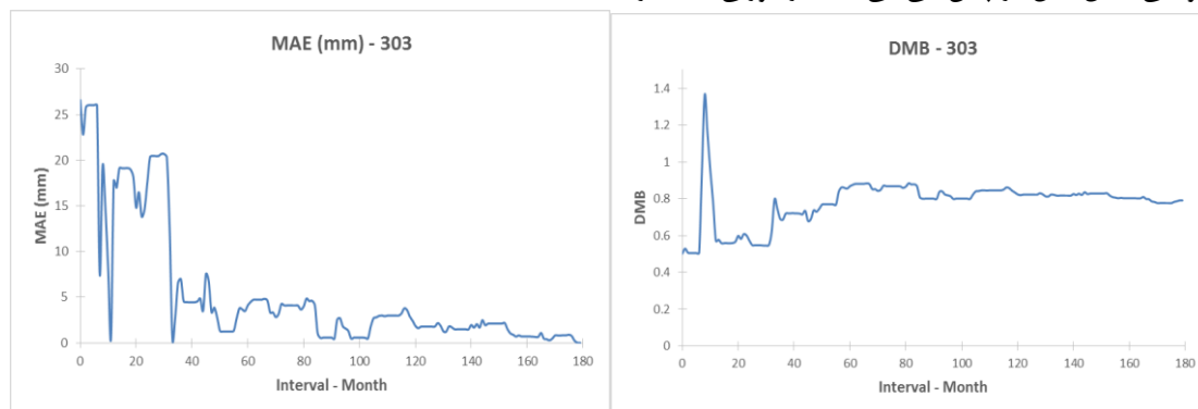
Fig. 3-Degree of mass balance (reight) and absolute error (left) in grid KB303 شکل ۳- میانگین درجه موازنه جرم (راست) و خطای مطلق (چپ) بارش سالانه برای شبکه KB303
