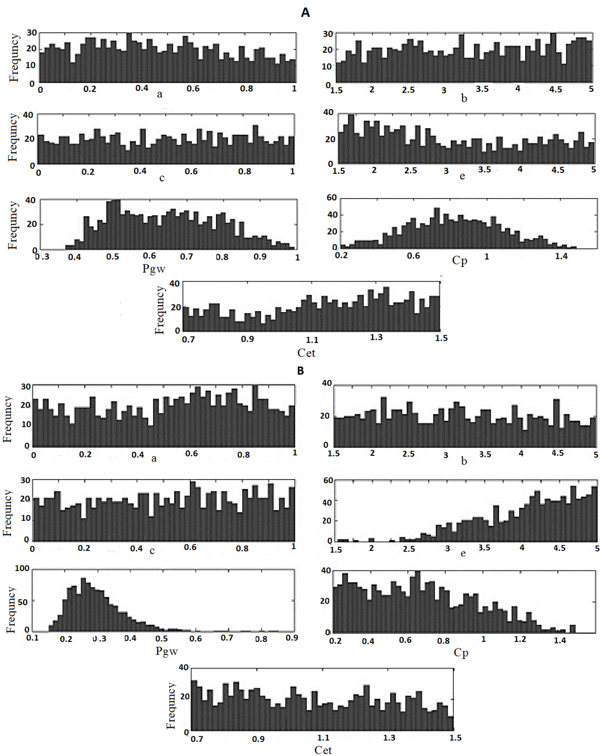
Fig. 4- The posterior distribution of SDDWB model parameters in the study areas A) Neyshabur B) Rokh شکل ۴- توزیع پسین پارامترهای مدل SDDWB در محدوده‌های مطالعاتی (A) نیشابور (B) رخ
