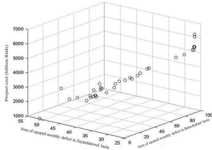
Fig. 12- Pareto front derived by the MOMCPSO-ANN-WEAP model (adaptive meta-model) شکل ۱۲- جبهه پرتو حاصل از مدل MOMCPSO-ANN-WEAP (فرامدل تطبیقی)
