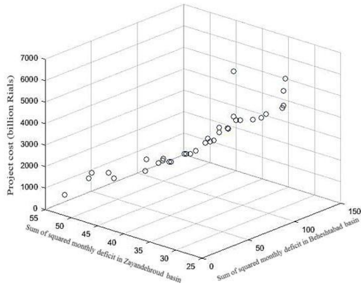
Fig. 11- Pareto front driven by the MOMCPSO-ANN model (sequential meta-model) شکل ۱۱- جبهه پرتو حاصل از مدل MOMCPSO-ANN (فرامدل ترتیبی)
