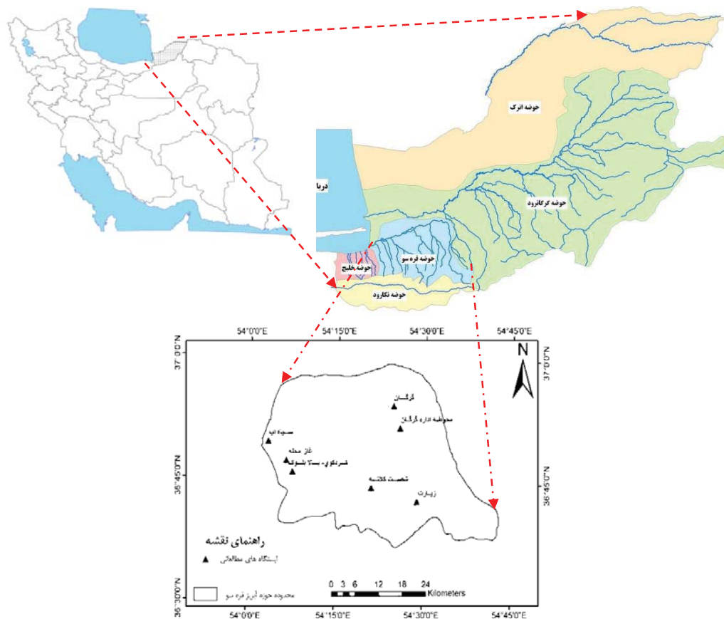
شکل ۱- موقعیت حوضه آبریز قره‌سو بر گستره ایران
