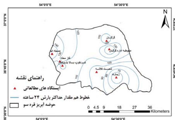
شکل ۳- خطوط هم مقدار PMP_{24} در حوضه آبریز قره سو
