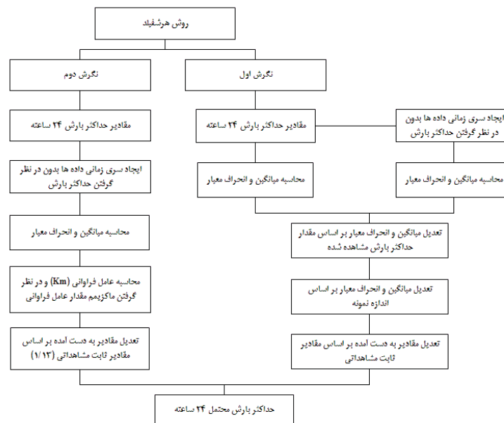
شکل ۲- فلوچارت روش هرشفیلد به منظور برآورد حداکثر بارش محتمل ۲۴ ساعته
