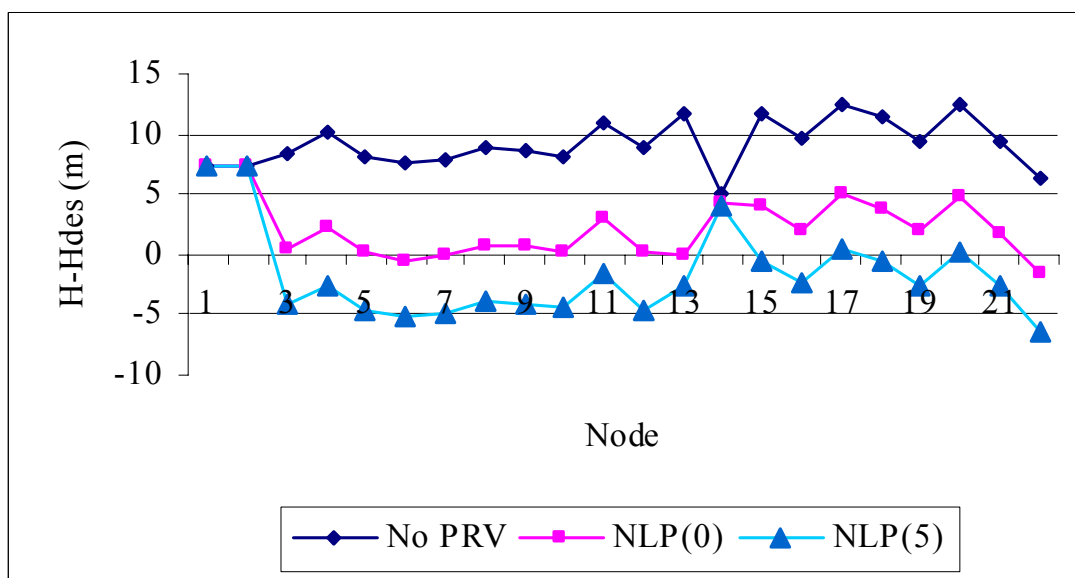
شکل ۷ - مقدار فشار اضافی در هر گره به ازای سناریوهای بدون شیر فشارشکن (No PRV)، شیر فشارشکن با \epsilon = 0 m، شیر فشارشکن با \epsilon = 5 m (NLP(0)) و \epsilon = 5 m (NLP(5)).
