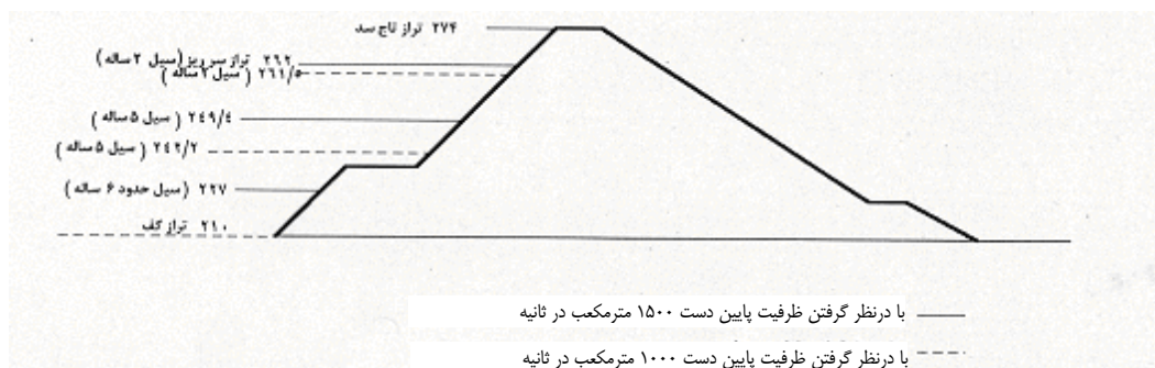
شکل ۱۰- درجه بندی مخزن سد پیشین
