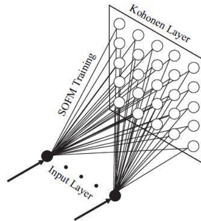
شکل ۱- طرح نمادین نگاشت مشخصه‌ی خود سازمانده کوهون؛ لایه‌ی ورودی شامل ویژگی‌های تجدید مقیاس شده‌ی حوضه‌ی آبریز است. (Rao and Srinivas, 2008)
