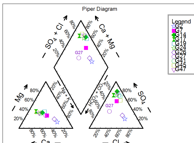
Fig. 7- Piper diagram of the Gotvand aquifer groundwater samples شکل ۷- نمودار پایپر نمونه‌های آب زیرزمینی آبخوان گنوند
